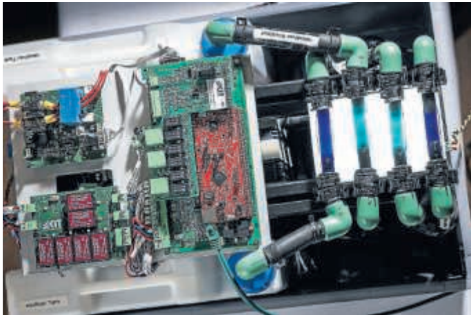
Das am KIT entwickelte Batterie-Management zum dezentralen Überwachen und Regeln von Redox-Flow-Batterien macht einen einfachen „stand alone“-Betrieb möglich. Foto: Markus Breig, KIT
